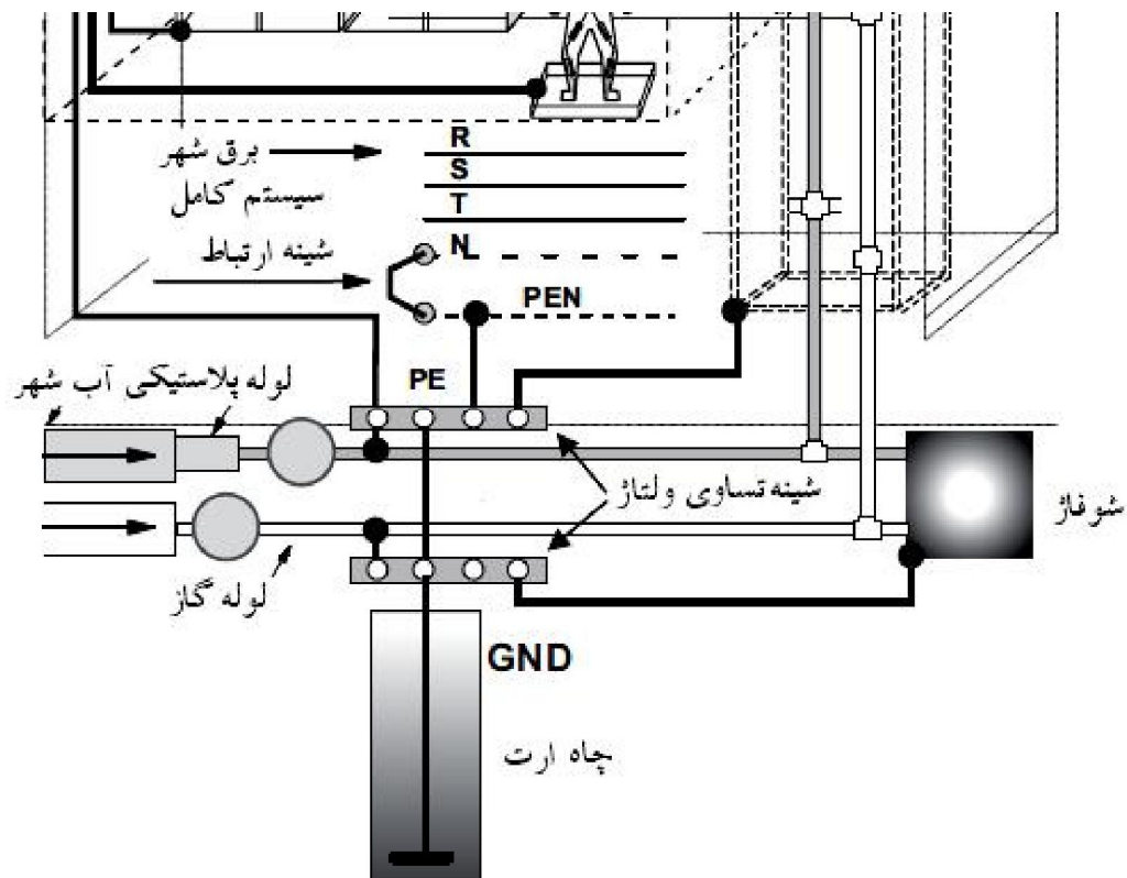
شکل ۶ سیستم کامل
